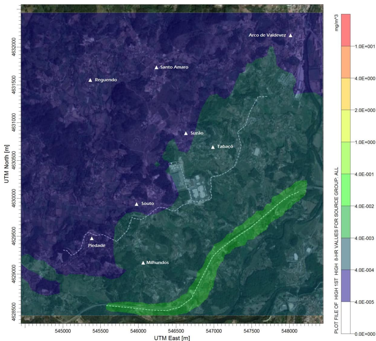
Figura 62 – Campo estimado das concentrações máximas das médias octohorárias de CO ( \text{mg.m}^{-3} ) verificadas no domínio em análise (Situação Actual).
