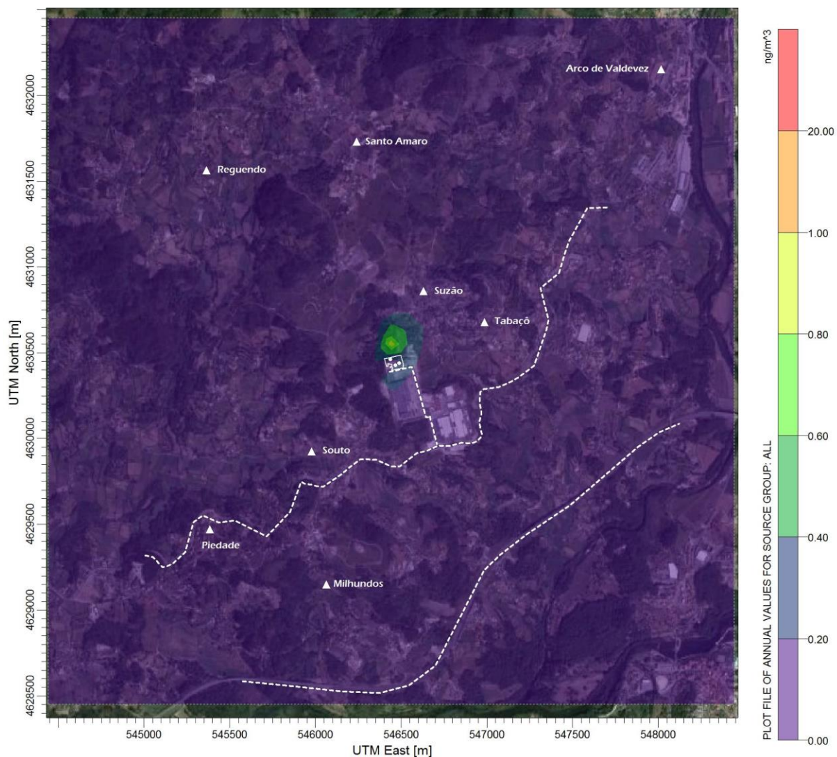
Figura 70 – Campo estimado das concentrações médias anuais de Ni ( \text{ng.m}^{-3} ) verificadas no domínio em análise (Situação Actual).
