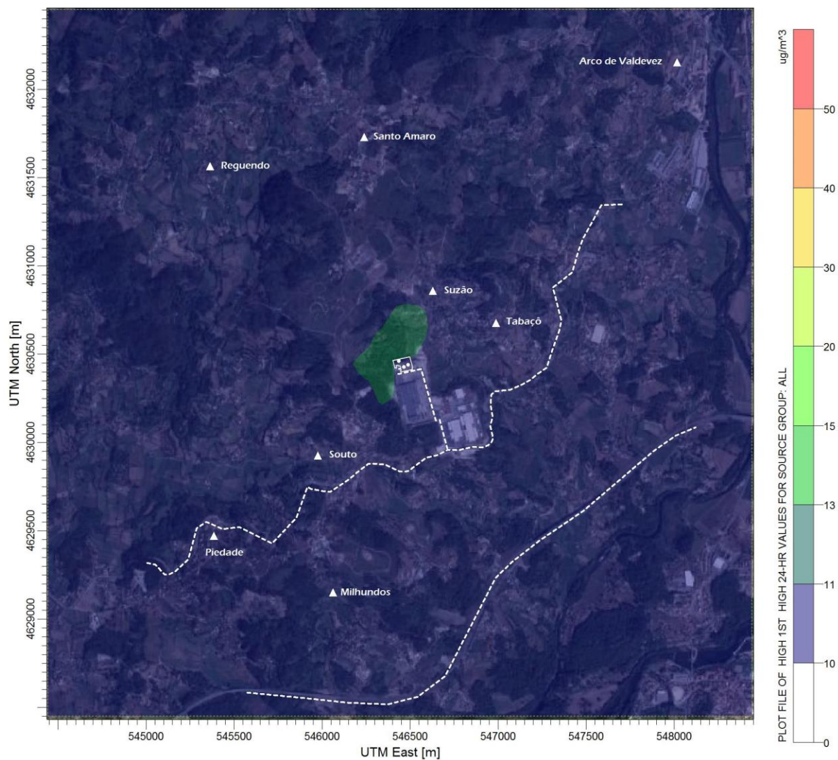
Figura 200 – Campo estimado das concentrações máximas das médias diárias de PM10 ( \mu\text{g.m}^{-3} ) verificadas no domínio em análise (Situação Futura).
