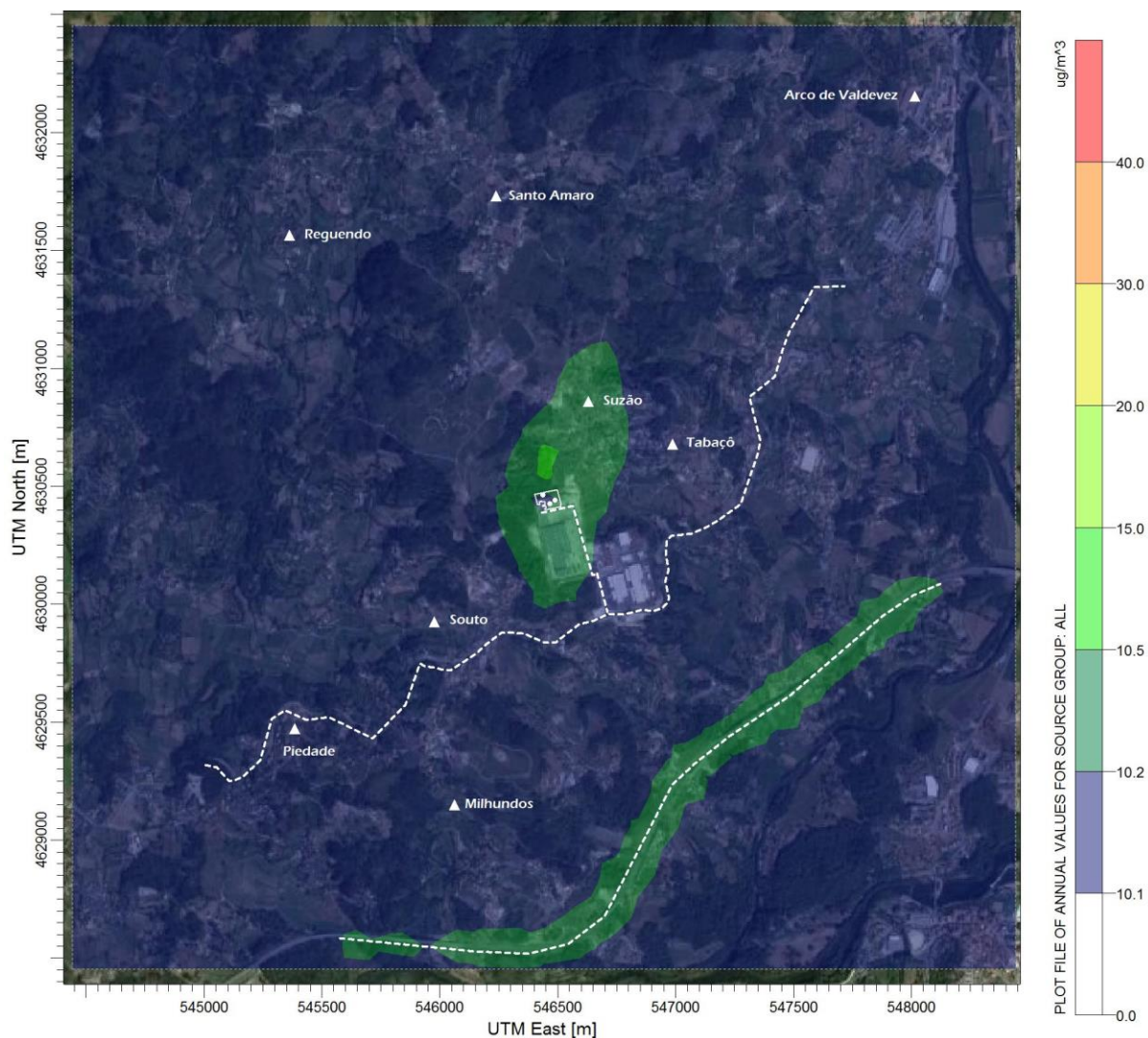
Figura 64 – Campo estimado das concentrações médias anuais de PM10 ( \mu\text{g.m}^{-3} ) verificadas no domínio em análise (Situação Actual).
