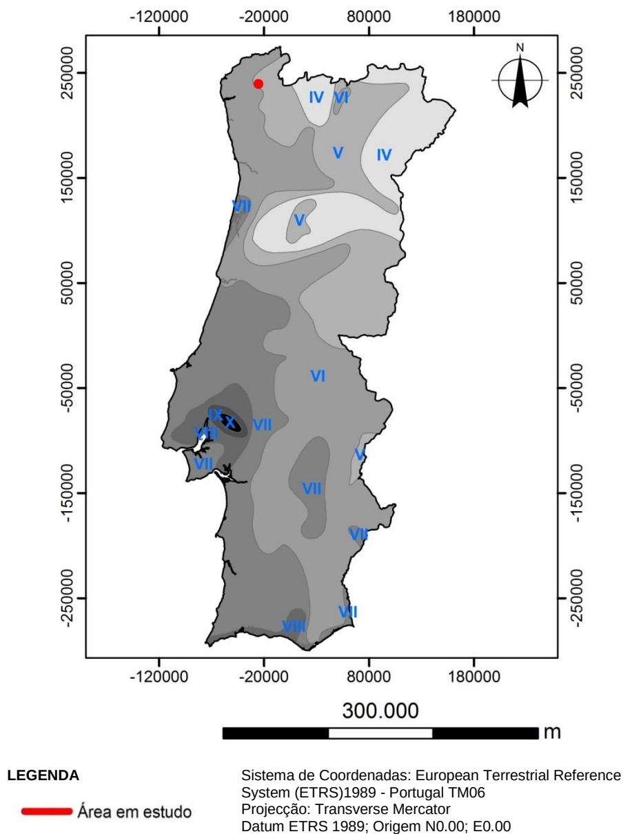
Figura 22 – Carta de intensidades sísmicas máximas.
