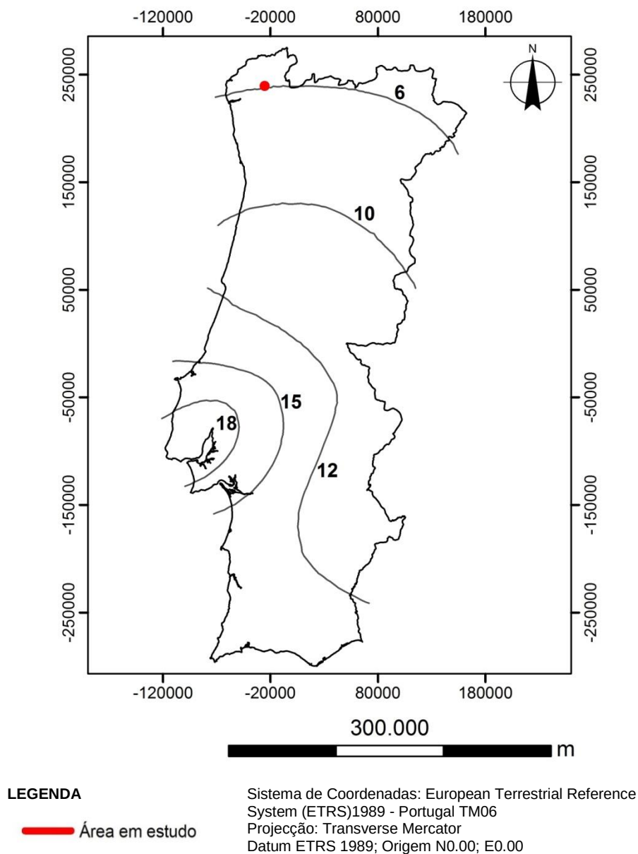
Figura 24 – Carta de isolinhas de velocidade máxima.
