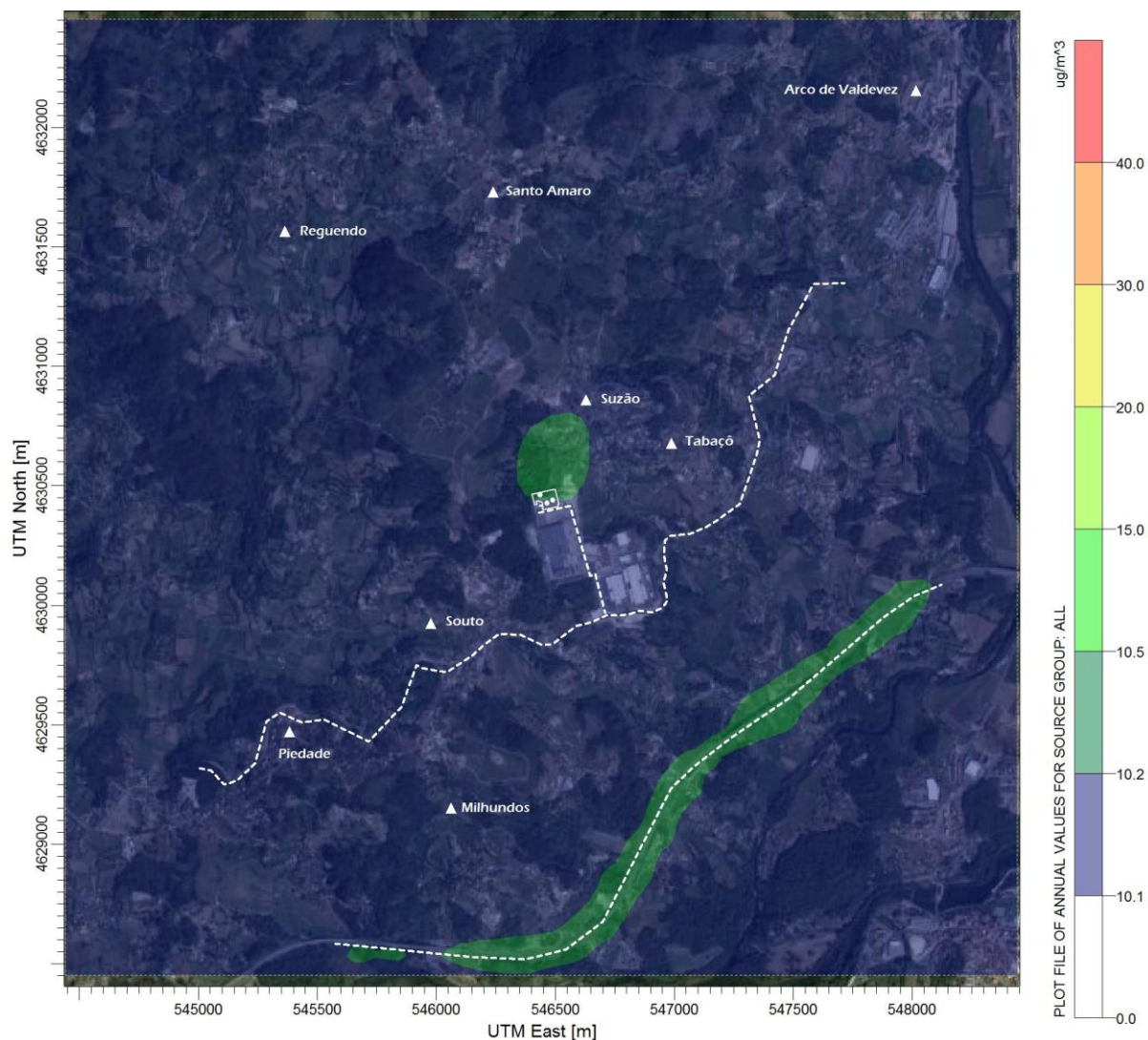
Figura 201 – Campo estimado das concentrações médias anuais de PM10 ( \mu\text{g.m}^{-3} ) verificadas no domínio em análise (Situação Futura).
