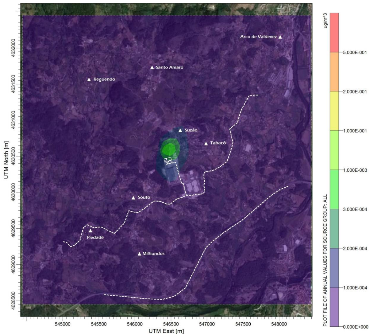
Figura 67 – Campo estimado das concentrações médias anuais de Pb ( \mu\text{g.m}^{-3} ) verificadas no domínio em análise (Situação Actual).
