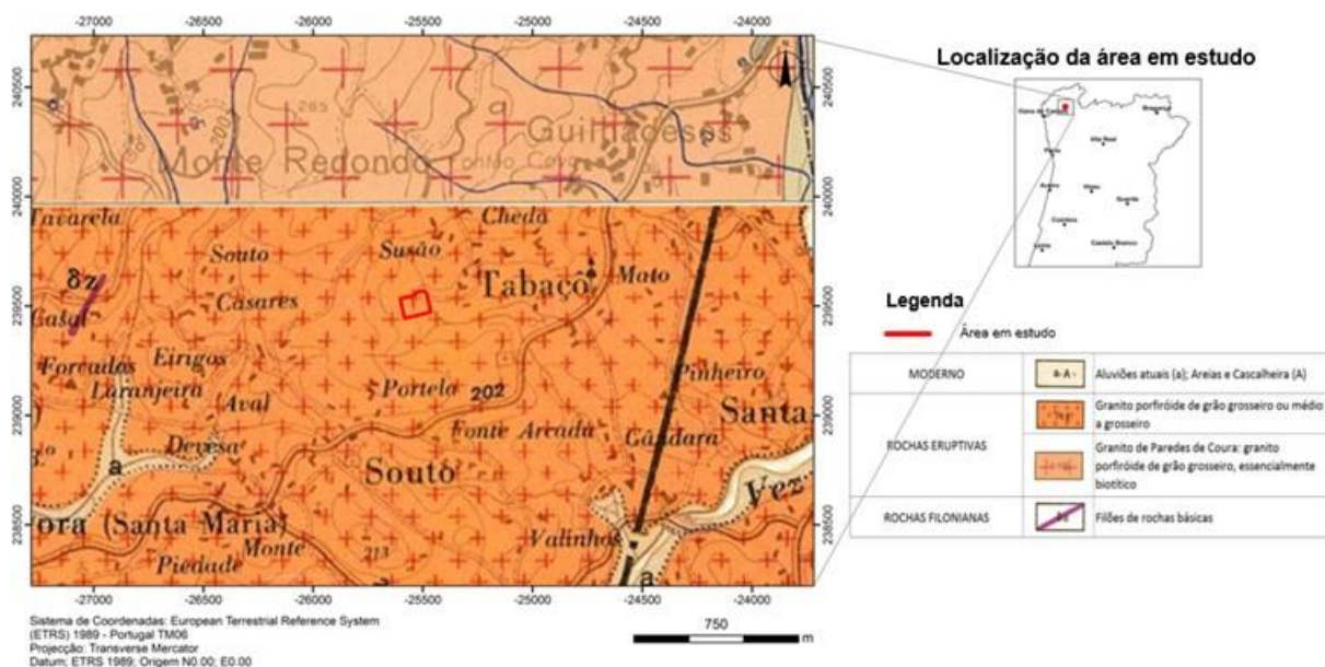
Figura 14 – Carta geológica.
