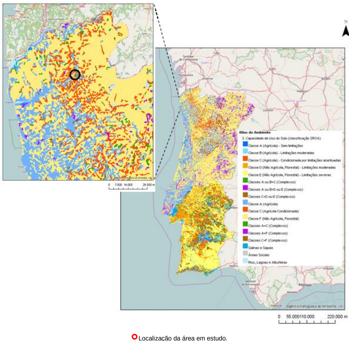
Figura 90 – Capacidade de Uso do Solo (classificação SROA (Serviço de Reconhecimento e Ordenamento Agrário))
