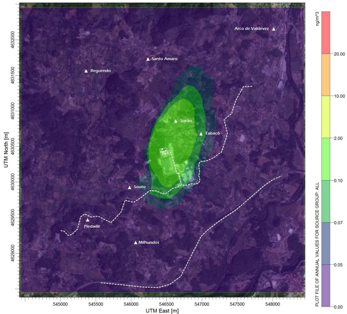
Figura 207 – Campo estimado das concentrações médias anuais de Ni ( \text{ng.m}^{-3} ) verificadas no domínio em análise (Situação Futura).
