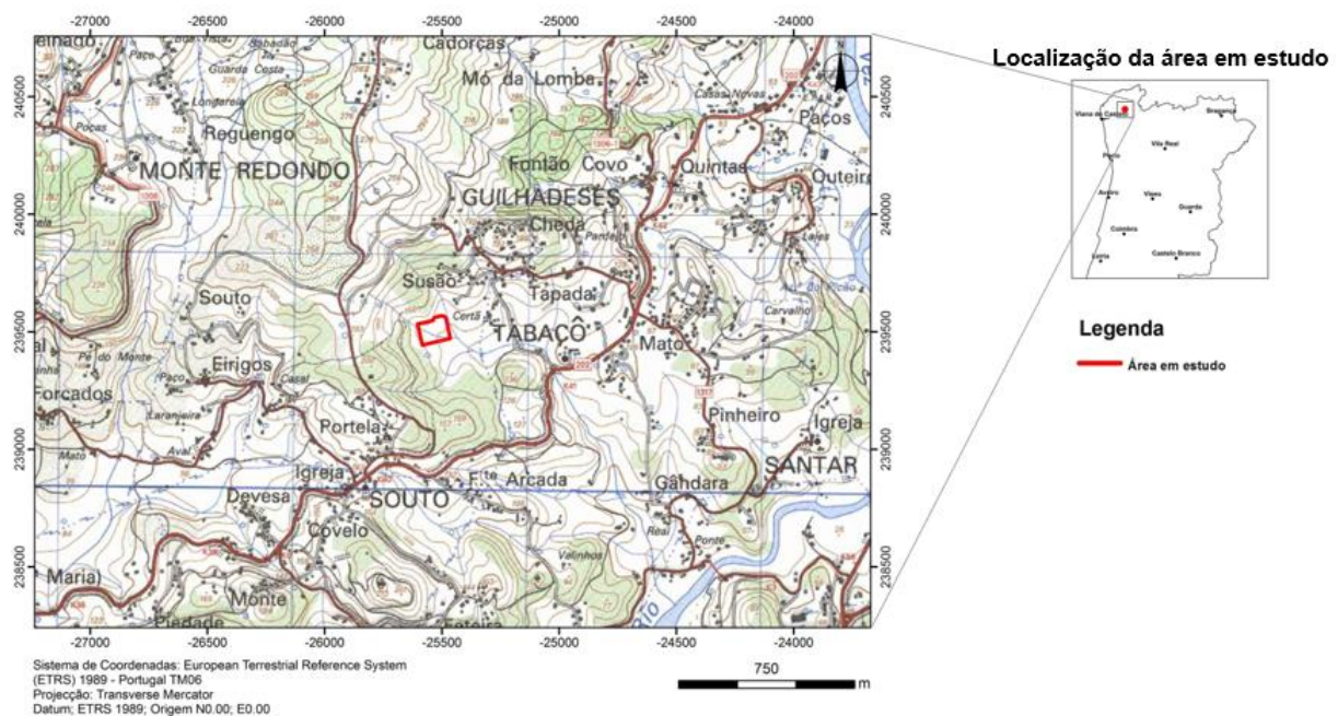
Figura 12 – Carta topográfica.
