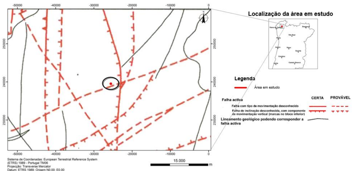
Figura 20 – Carta neotectónica
