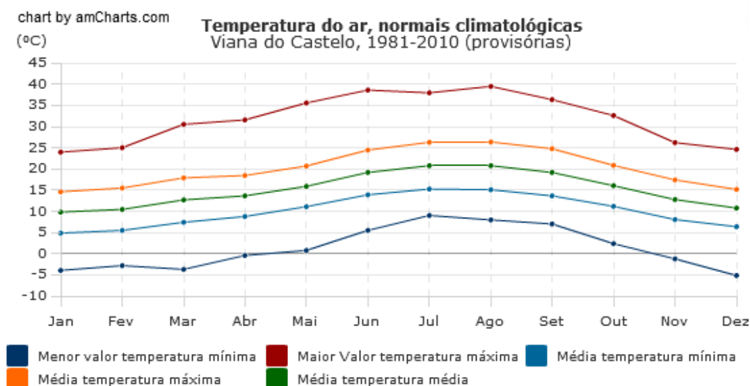
Figura 187 - Variação anual dos principais parâmetros da temperatura do ar, para a estação climatológica de Viana do Castelo, no período de 1981 a 2010.
