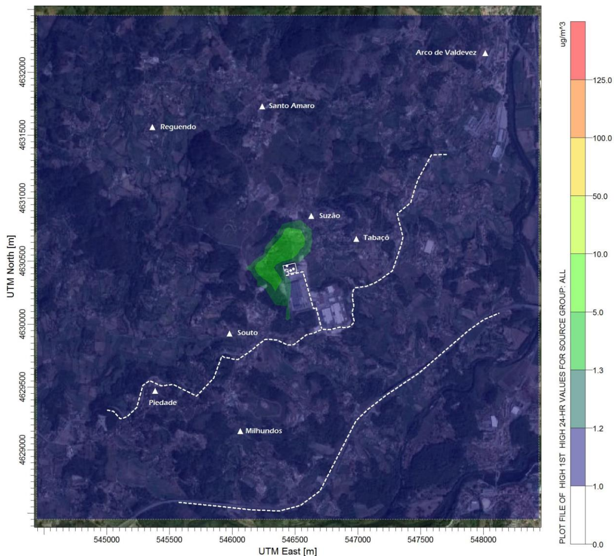
Figura 203 – Campo estimado das concentrações máximas das médias diárias de SO 2 (µg.m -3 ) verificadas no domínio em análise (Situação Futura).
