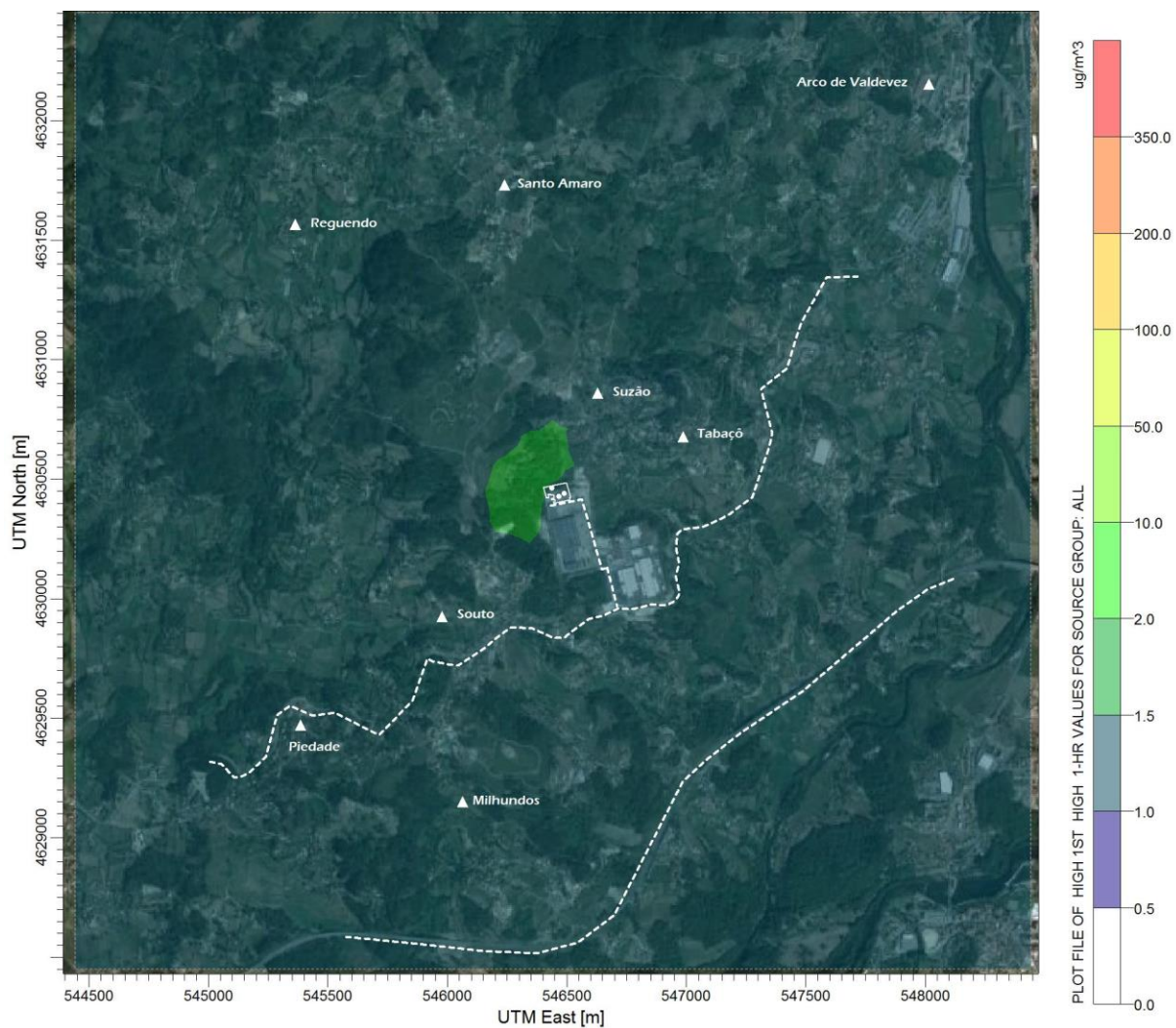
Figura 65 – Campo estimado das concentrações máximas das médias horárias de SO 2 (µg.m -3 ) verificadas no domínio em análise (Situação Actual).
