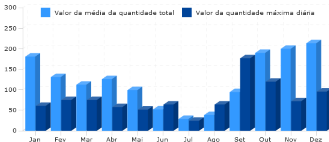
Figura 190 – Variação média da precipitação na estação climatológica de Viana do Castelo, no período de 1981-2010.
