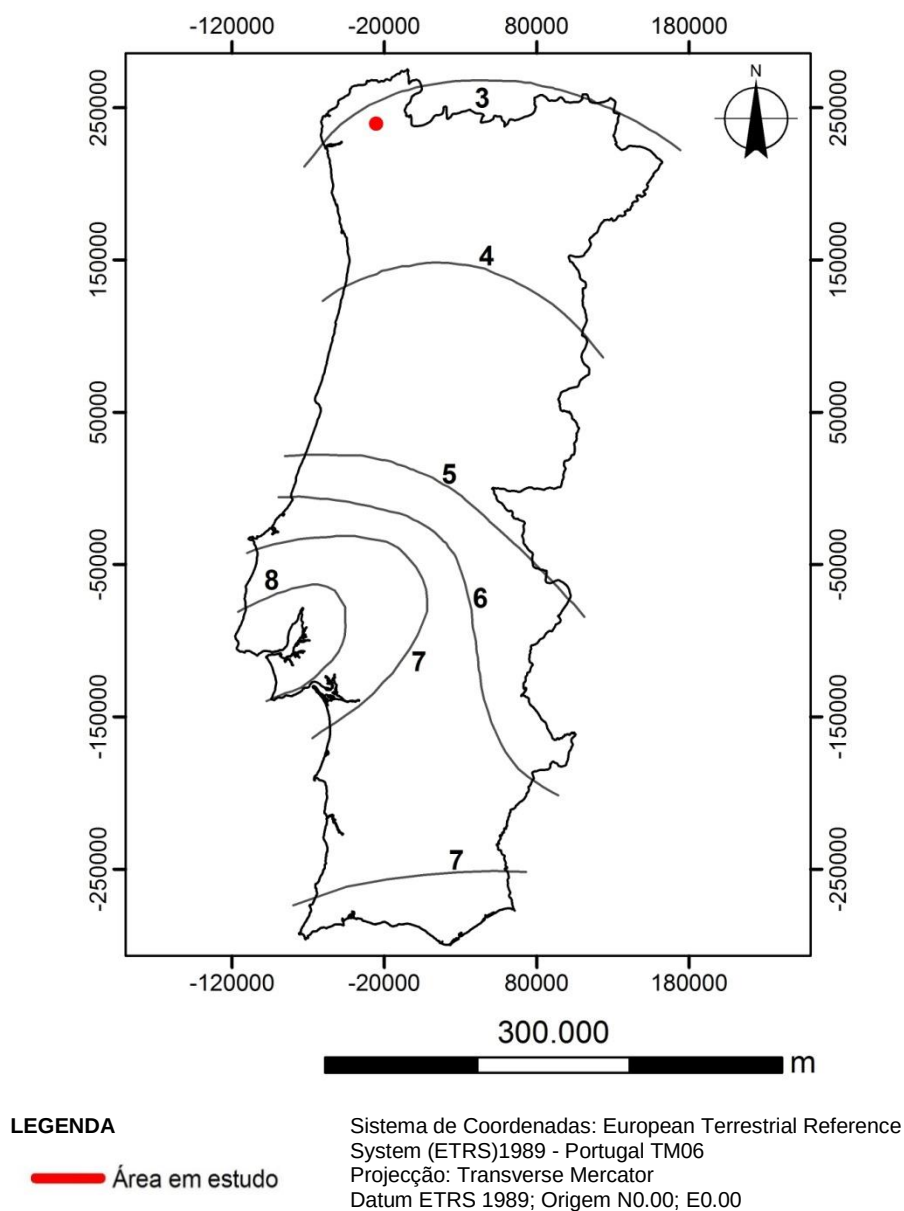
Figura 25 – Carta de isolinhas de deslocamento máximo.
