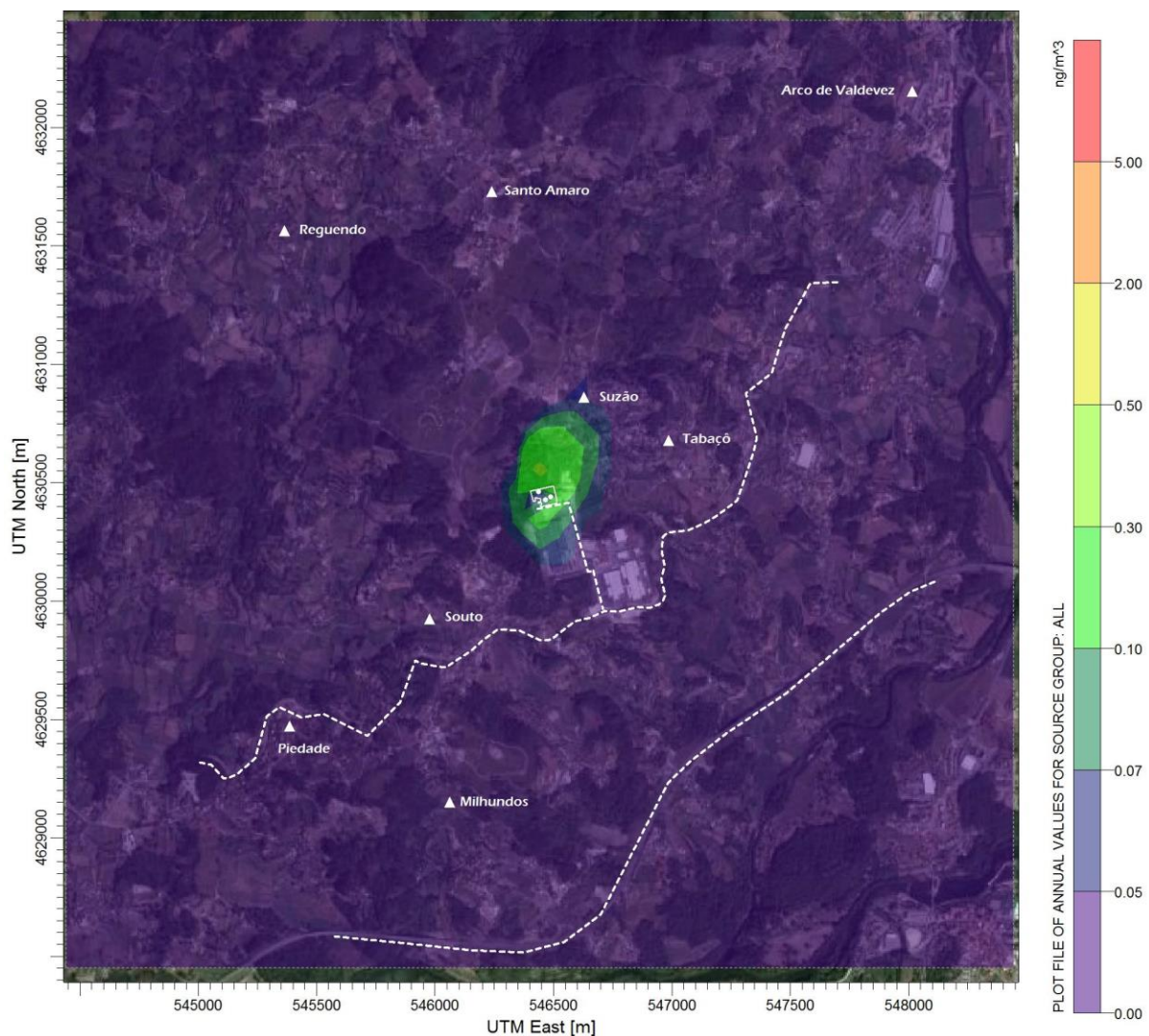
Figura 69 – Campo estimado das concentrações médias anuais de Cd ( \text{ng.m}^{-3} ) verificadas no domínio em análise (Situação Actual).
