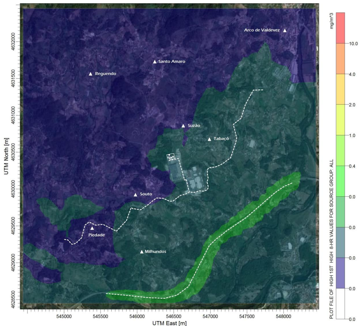
Figura 199 – Campo estimado das concentrações máximas das médias octohorárias de CO ( \text{mg.m}^{-3} ) verificadas no domínio em análise (Situação Futura).
