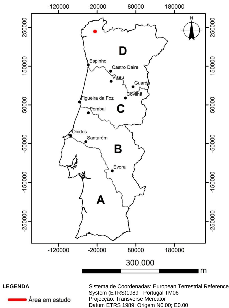
Figura 21 – Zonas sísmicas propostas pelo RSAEEP.
