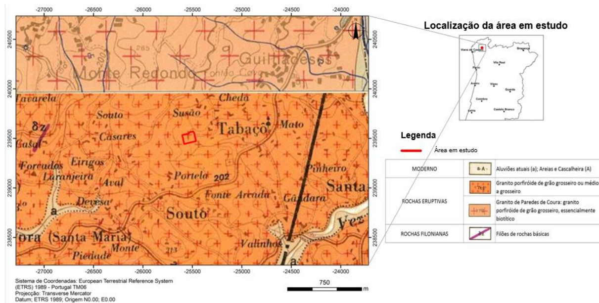
Figura 28 – Carta geológica
