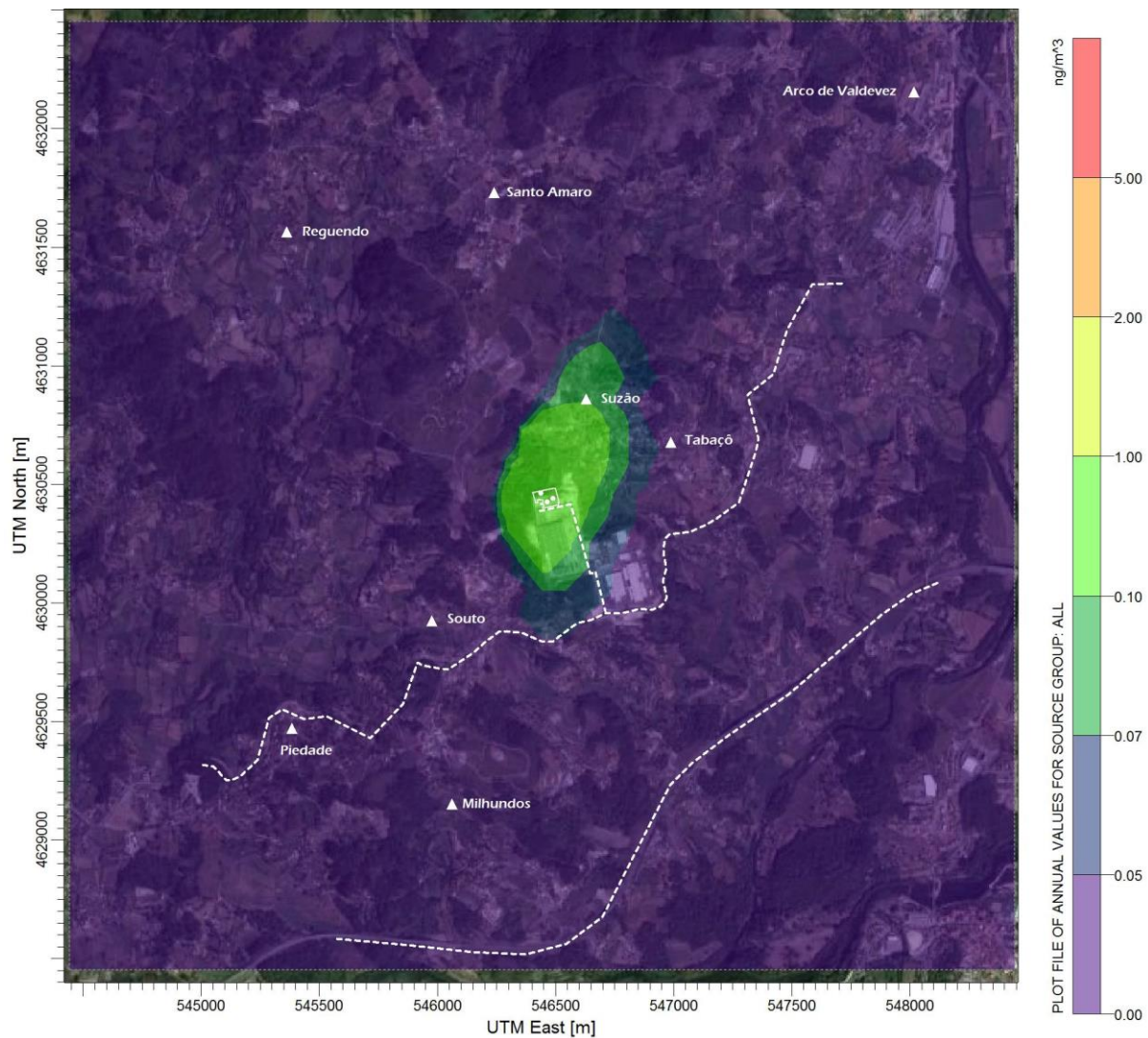
Figura 206 – Campo estimado das concentrações médias anuais de Cd (ng.m-3) verificadas no domínio em análise (Situação Futura).
