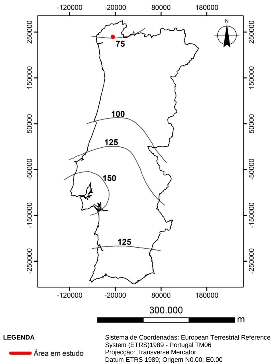
Figura 23 – Carta de isolinhas de aceleração máxima.
